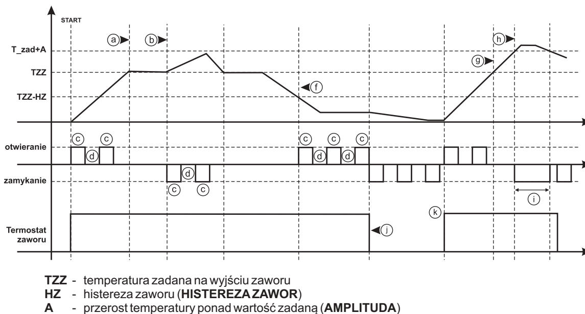
Rys.16. Praca zaworu w trybie normalnym z termostatem zaworu
