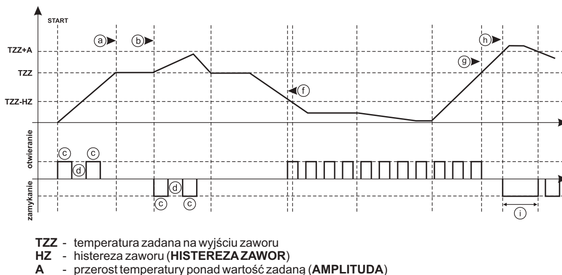
Rys.15. Praca zaworu w trybie normalnym z termostatem zaworu
