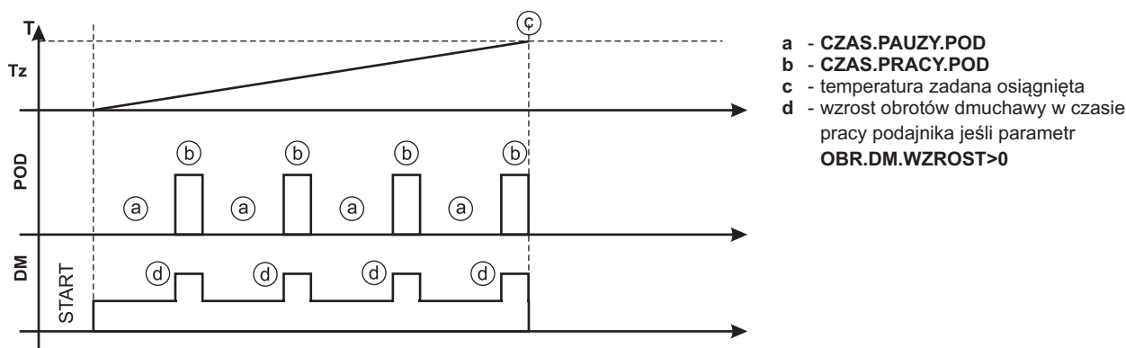
Rys.11. Interpretacja graficzna czasu pracy i czasu paazy podajnika.
