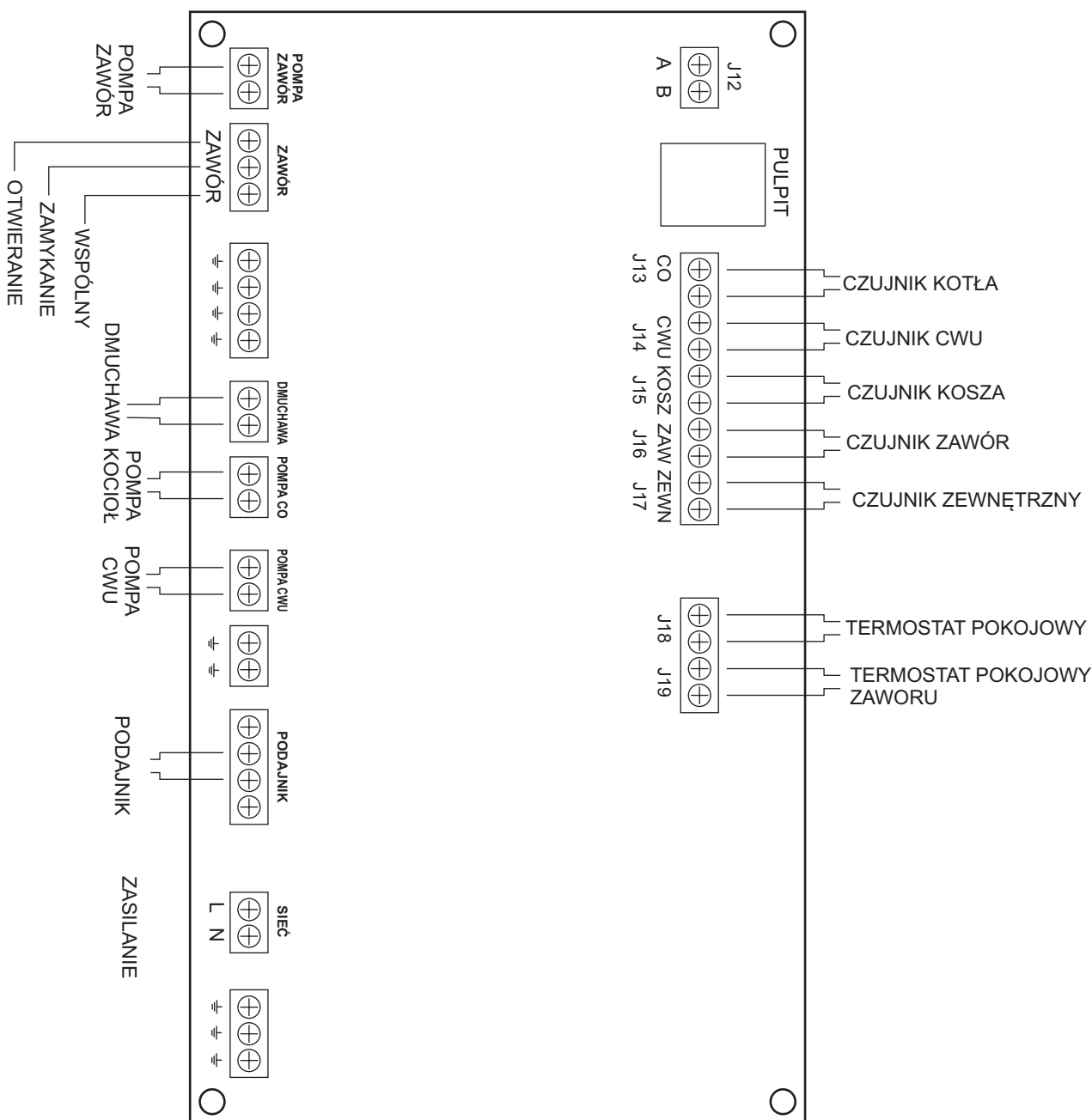
Rys.19. Widok płyty głównej z kostkami montażowymi do podłączenia urządzeń wejścia/wyjścia.
