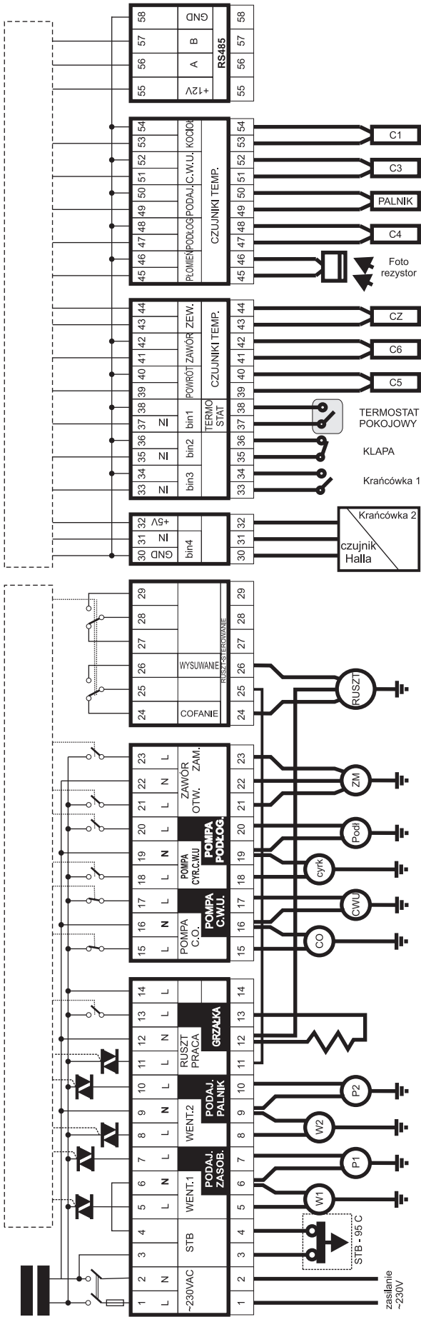
Sterownik Control TOUCH - PELLET schemat podłączeń elektrycznych
