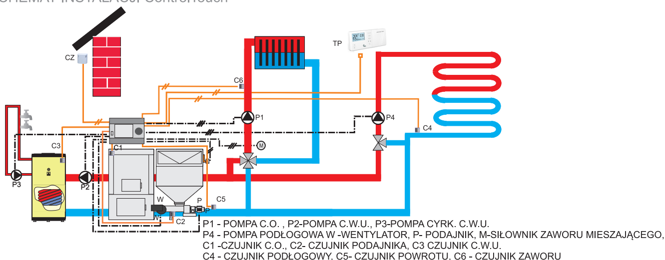
SCHEMAT INSTALACJI ControlTouch
