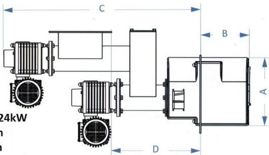
Rysunek nr 2. Wymiary palnika SV300
