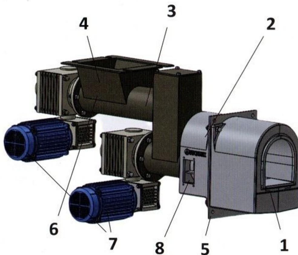
Rysunek nr 1. Budowa palnika
